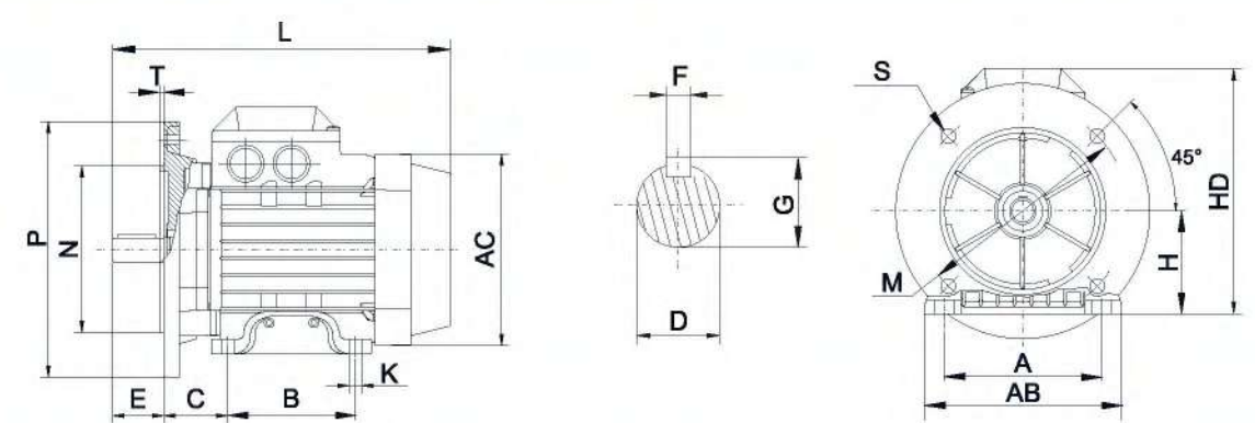
B35 卧立式大法兰两用安装80-180 ( IE2、IE3 ) 机座尺寸图
