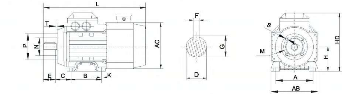
B34 卧式小法兰两用安装 63-112 机座尺寸图
