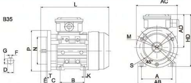
B35 卧式大法兰两用安装 63-180 机座尺寸图
