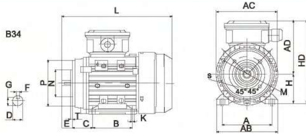
B34 卧式小法兰两用安装 63-112 机座尺寸图
