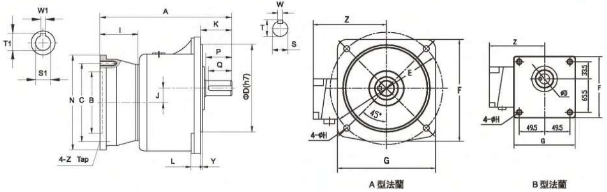
入力孔尺寸 Input Bore
