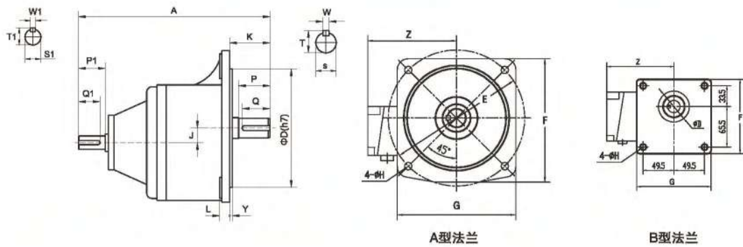
A型法蘭
