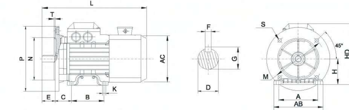
B35 卧式大法兰两用安装 63-180 机座尺寸图
